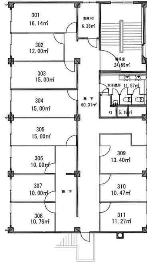
3階平面図
