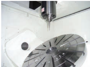
大型同時5軸制御 立形マシニングセンタ
