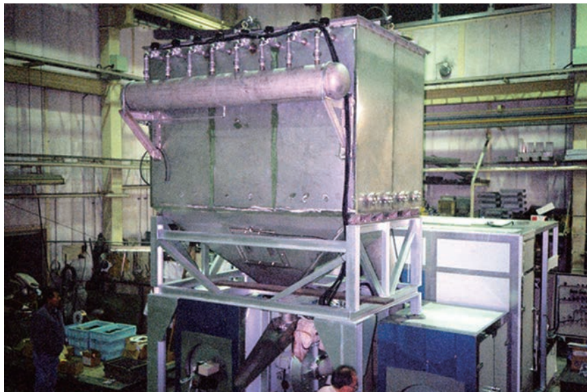
大型板金：電力会社の使用したコークスを粉末にし乾燥させ、湖水や川などを綺麗にする総ステン装置です。
