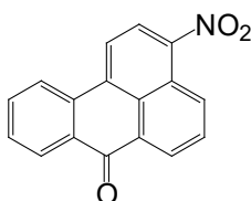
図1 3-ニトロベンズアントロン
