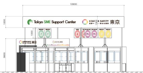
■ B.Elevation
