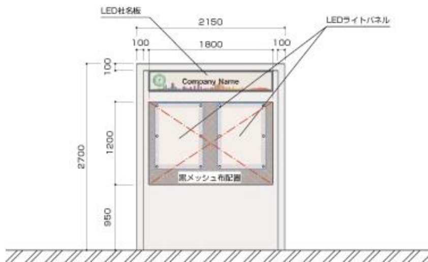
■ A.Elevation
