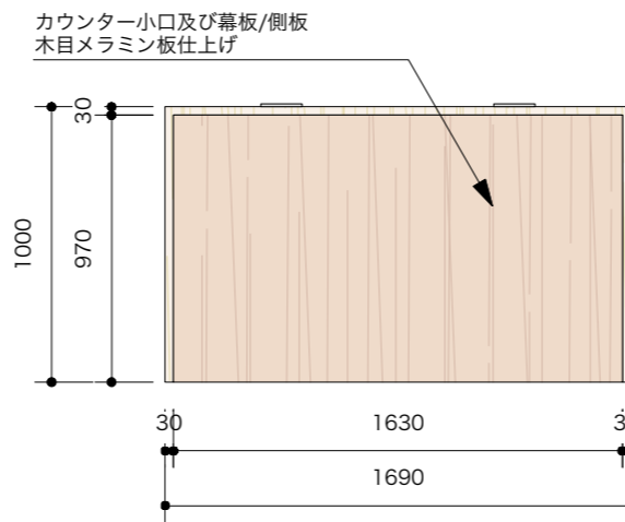
正面図
