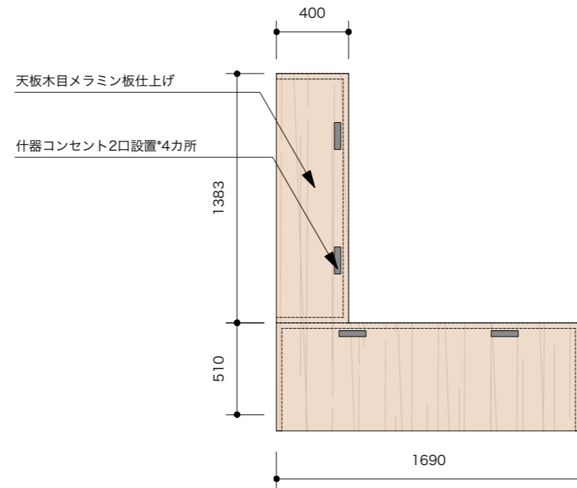
上面図
