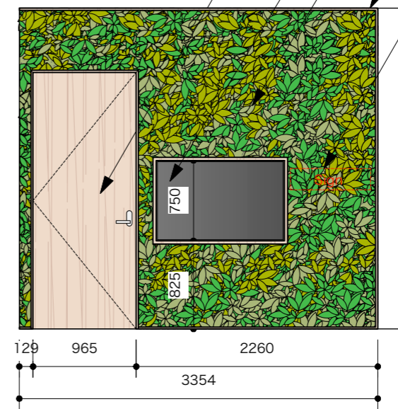
展開図C
