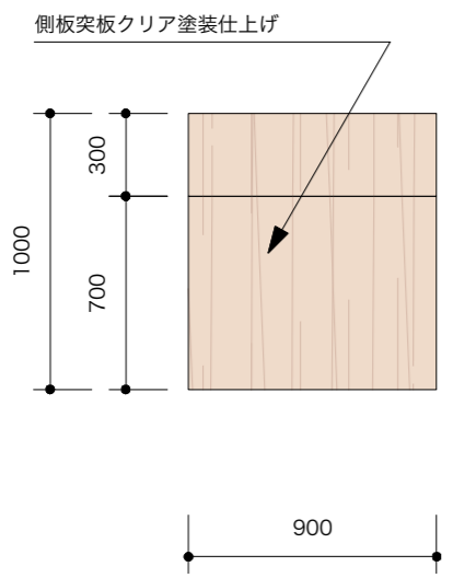
側面図
