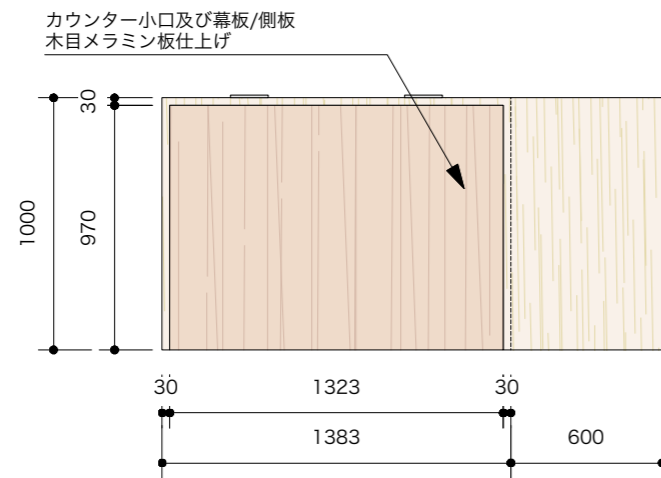
左側面図
