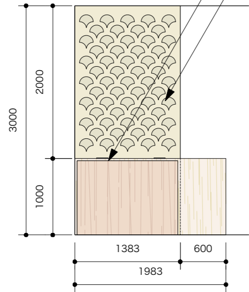
展開図A
