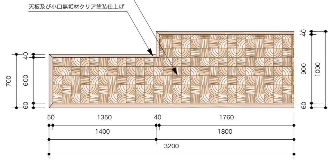
正面図
