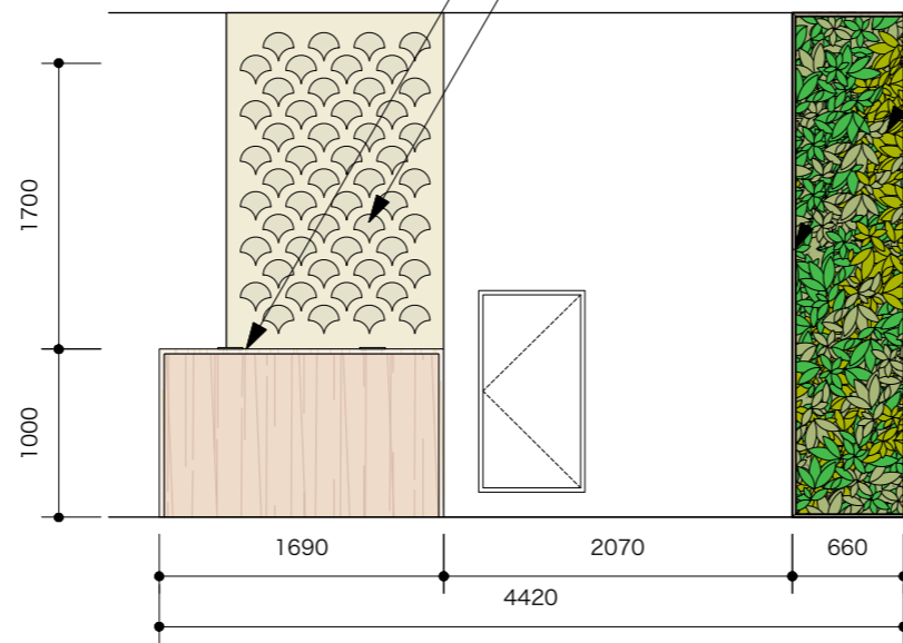
展開図B
