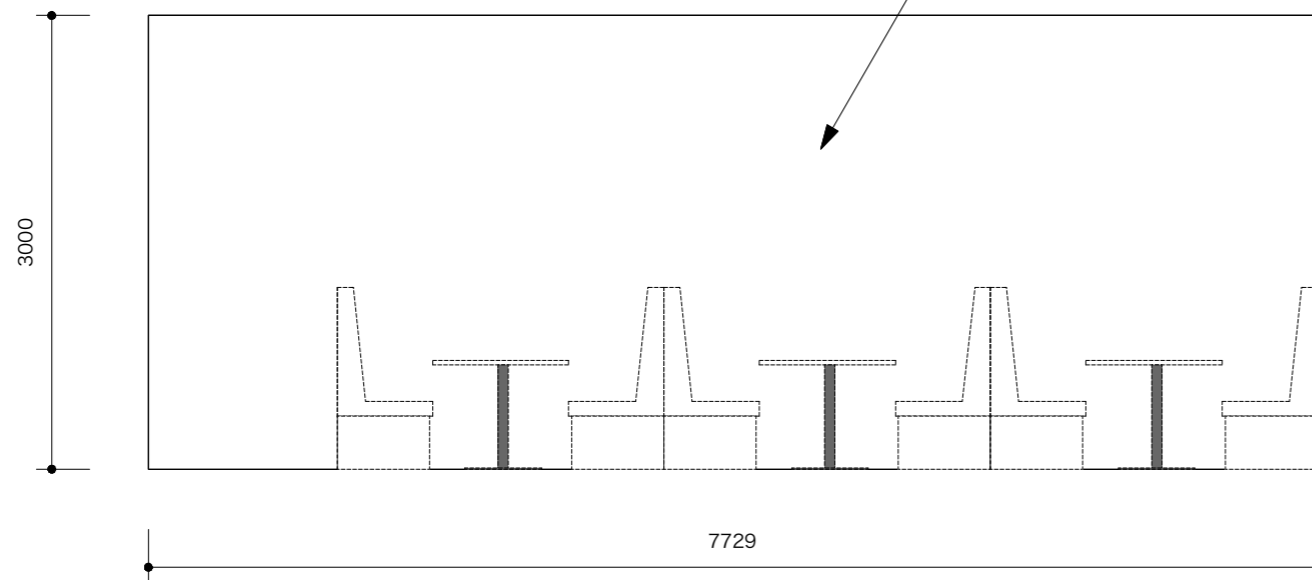
展開図D
