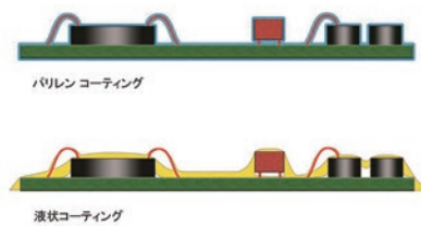
極薄かつ均一な膜厚のパリレンコーティング
