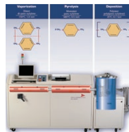
パリレン気相蒸着プロセス
