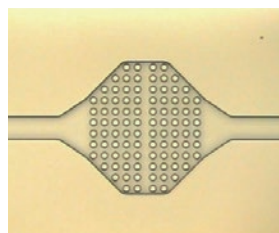
フォトレジストで μTAS 流路形成が可能
