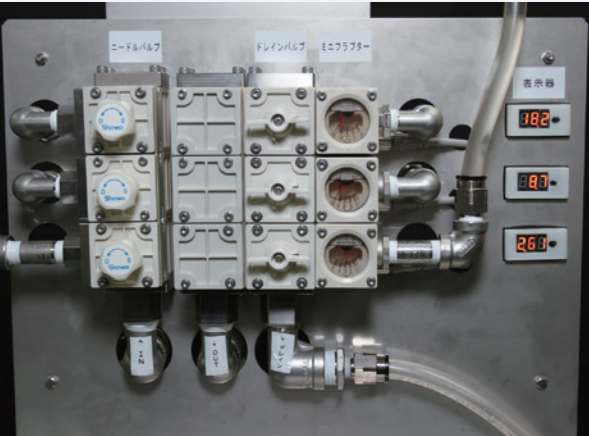
開発製品 小型流量計「ミニフラプターシリーズ」
