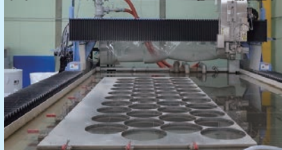
CFRP（炭素繊維強化プラスチック）カットの一例
