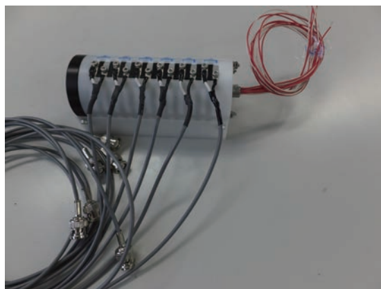
6極歪ゲージ対応ロータリーコネクタ
